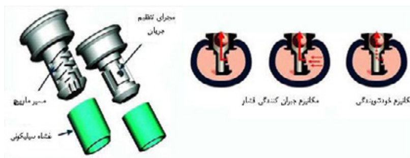
شکل ۲- جزئیات قطره چکان های مخصوص زیر سطح
